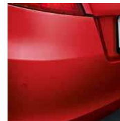
3.10 Датчики парковки. Комплект из 4 шт. с пьезоэлементами. Сенсоры могут быть окрашены в цвет кузова. Передние. 990E0-68L55-000 Задние. 990E0-68L53-015
